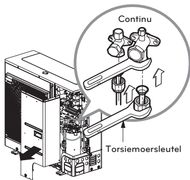
Eenheid buiten
