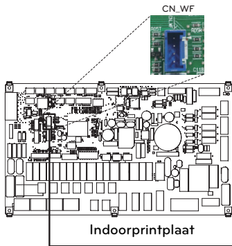
Indoorprintplaat
